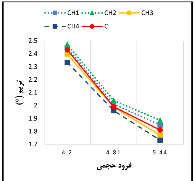
شکل ۲۱- نمودار تیریم شناورهای پروازی در مقایسه با هم در شبیه-سازی های عددی صورت گرفته در فرود حجمی ۴/۲، ۴/۸۱ و ۵/۴۴
