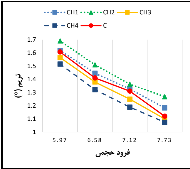
شکل ۲۲- نمودار تیریم شناورهای پروازی در مقایسه با هم در شبیه-سازی های عددی صورت گرفته در فرود حجمی ۵/۹۷، ۶/۵۸، ۷/۱۲ و ۷/۷۳
