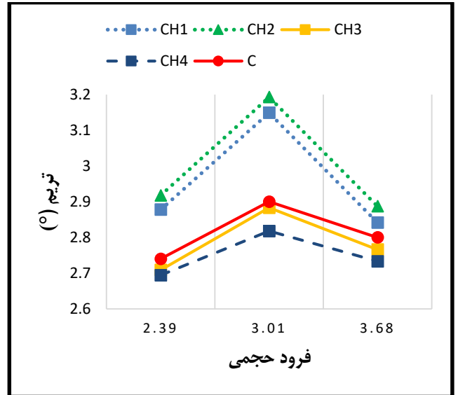
شکل ۲۰- نمودار تیریم شناورهای پروازی در مقایسه با هم در شبیه-سازی های عددی صورت گرفته در فرود حجمی ۲/۳۹، ۳/۰۱ و ۳/۶۸
